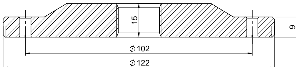
SEZIONE A-A
