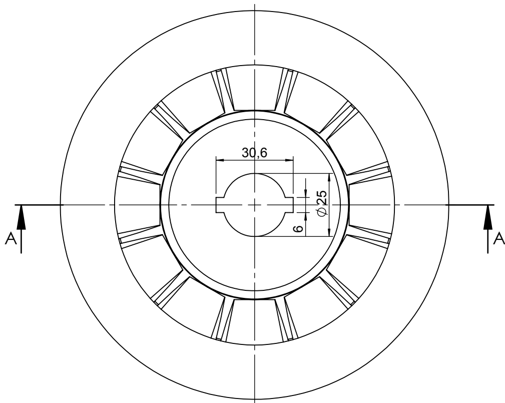
SEZIONE A-A
