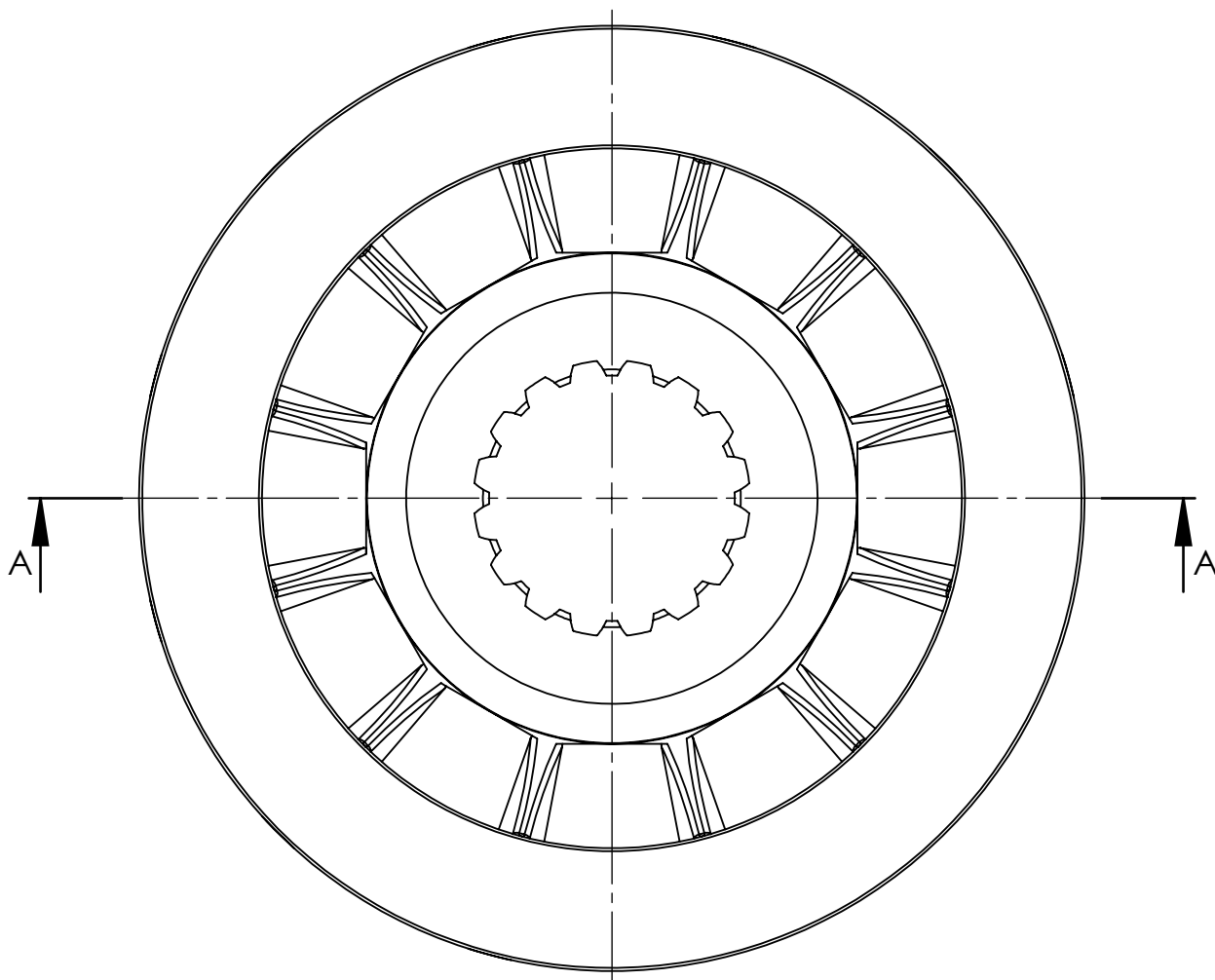
SEZIONE A-A
