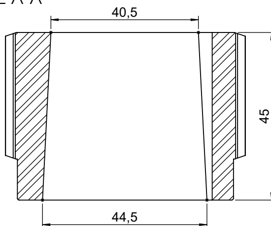
SEZIONE A-A
