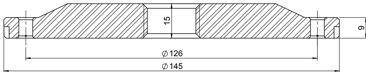
SEZIONE A-A
