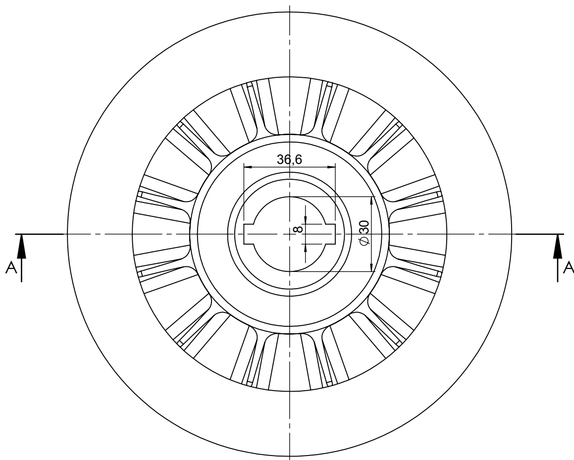
SEZIONE A-A
