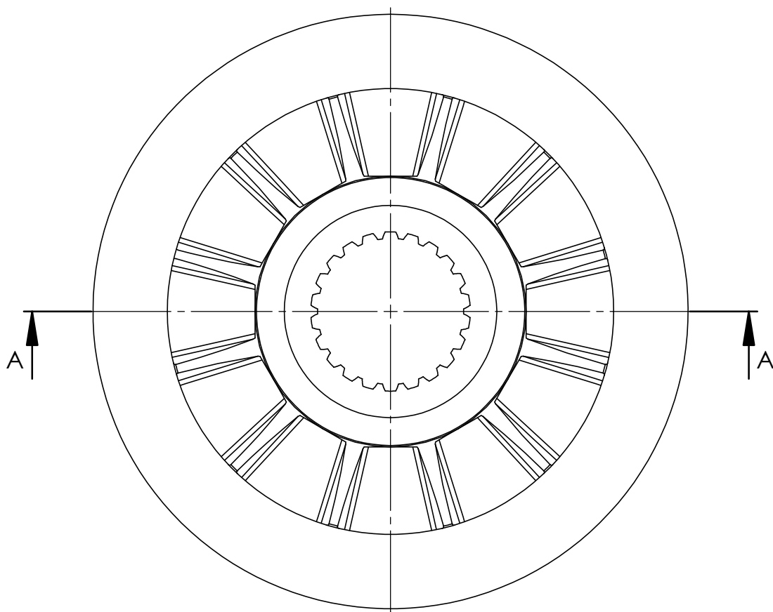
SEZIONE A-A
