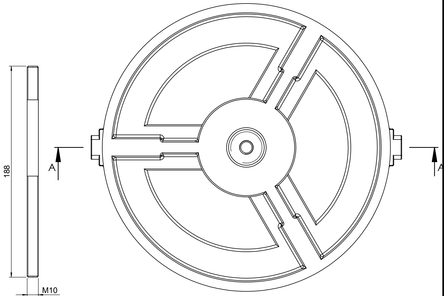
SEZIONE A-A
