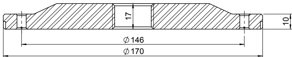
SEZIONE A-A
