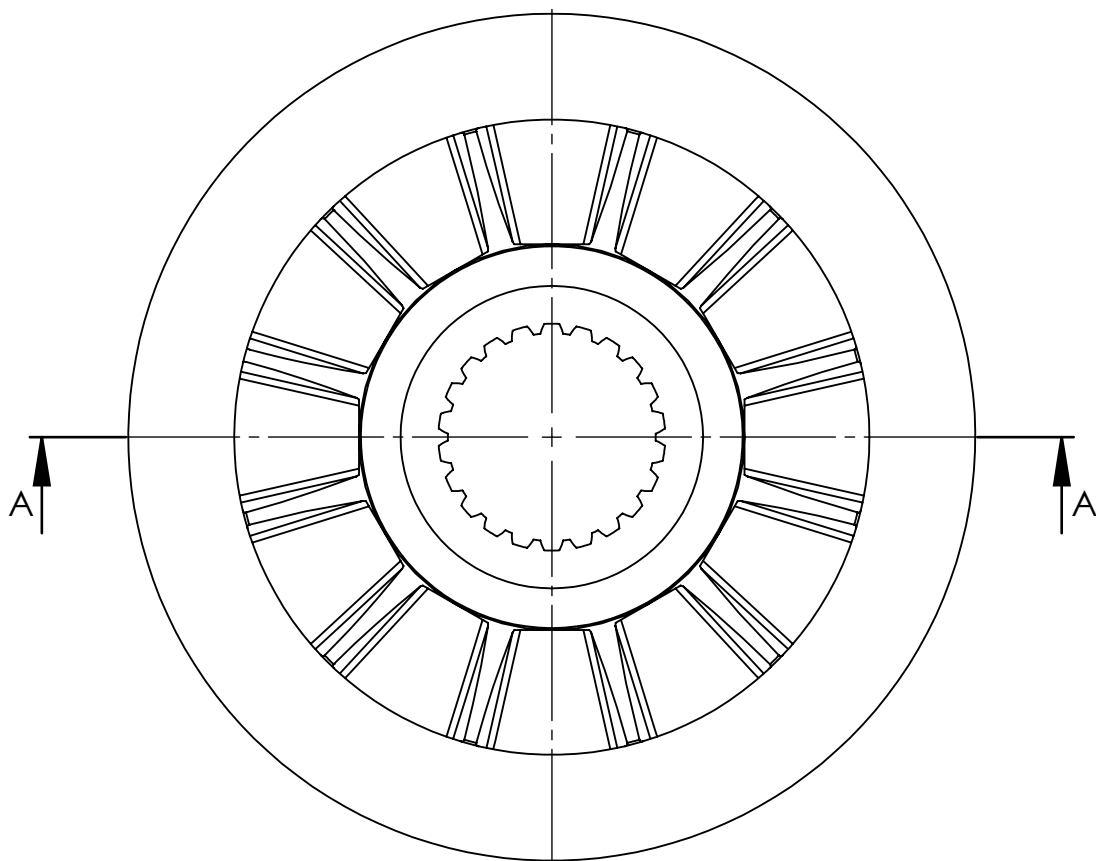
SEZIONE A-A
