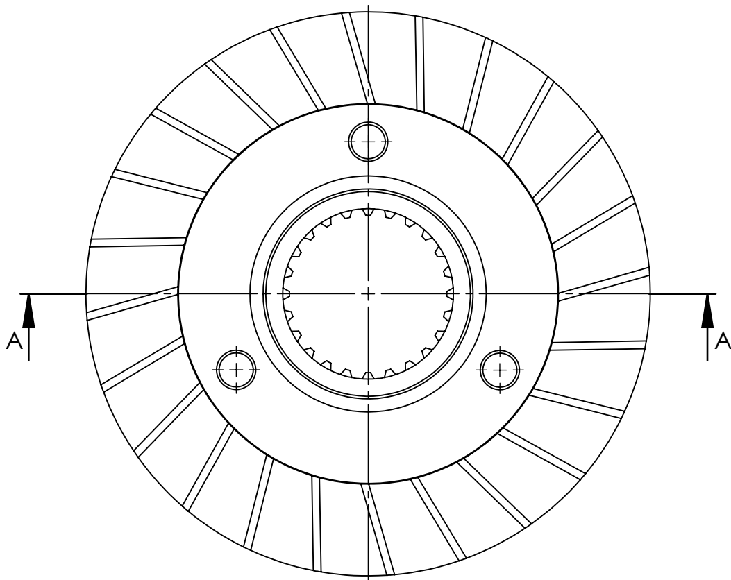
SEZIONE A-A
