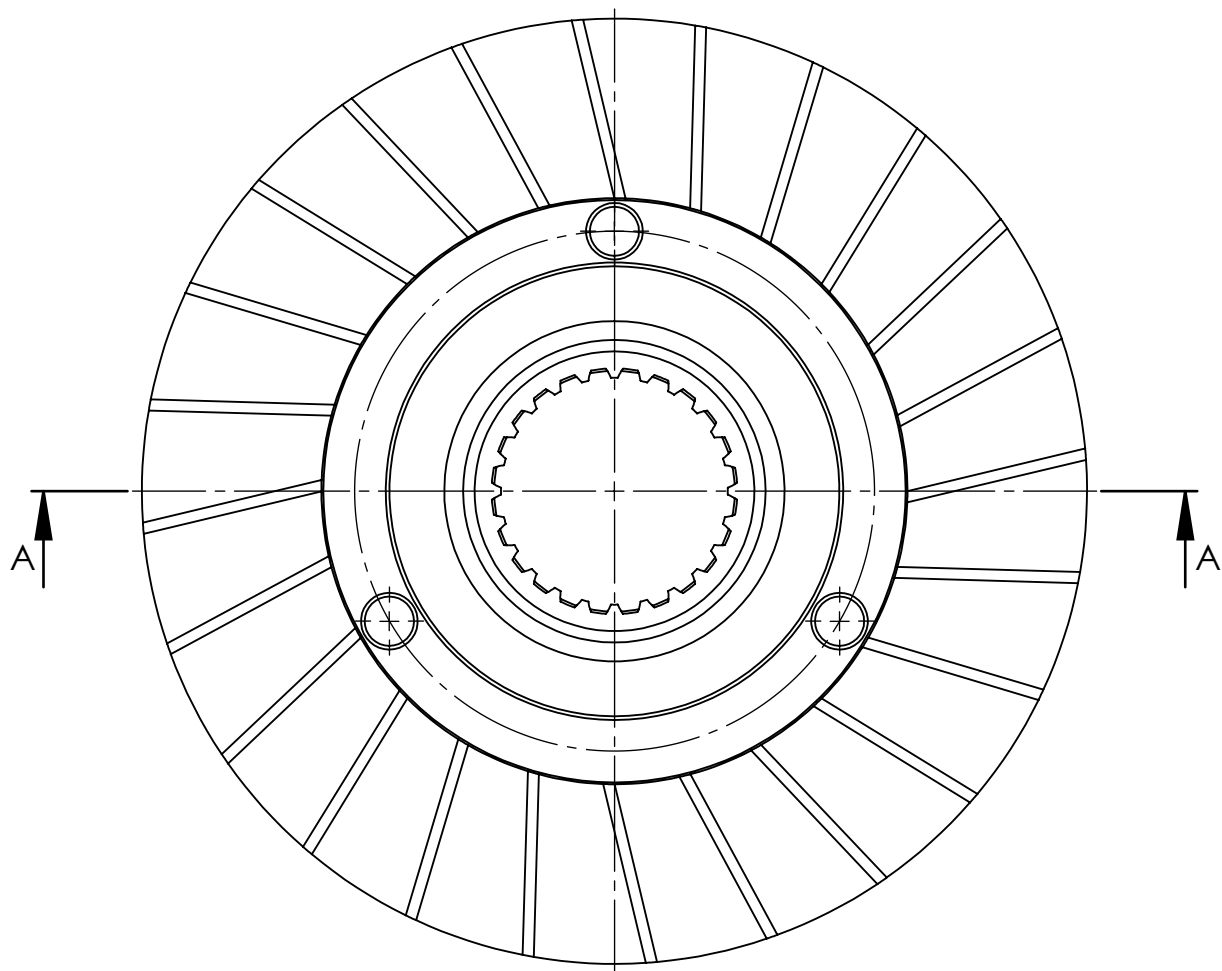
SEZIONE A-A
