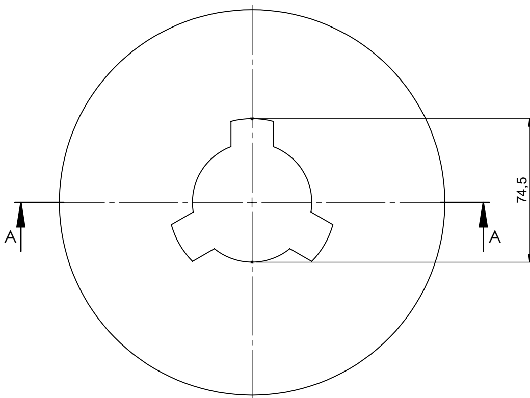
SEZIONE A-A
