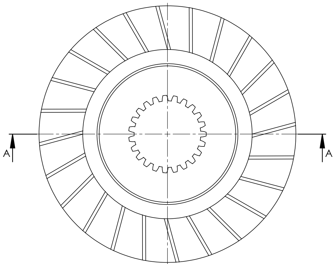
SEZIONE A-A
