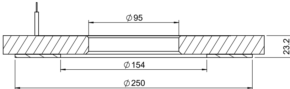
SEZIONE A-A
