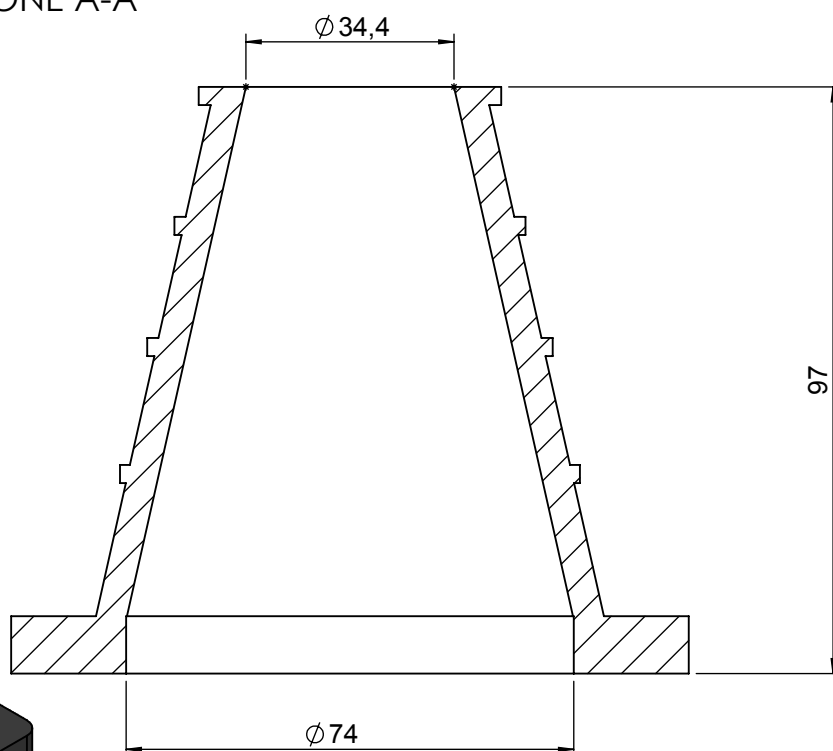
SEZIONE A-A
