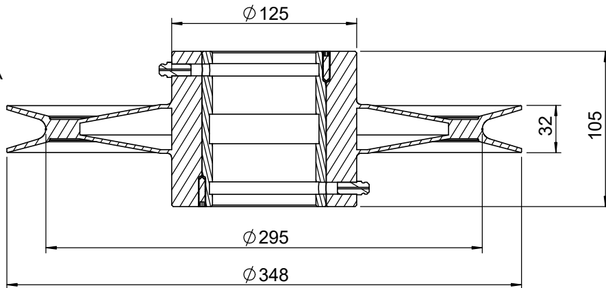
SEZIONE A-A
