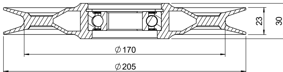
SEZIONE A-A
