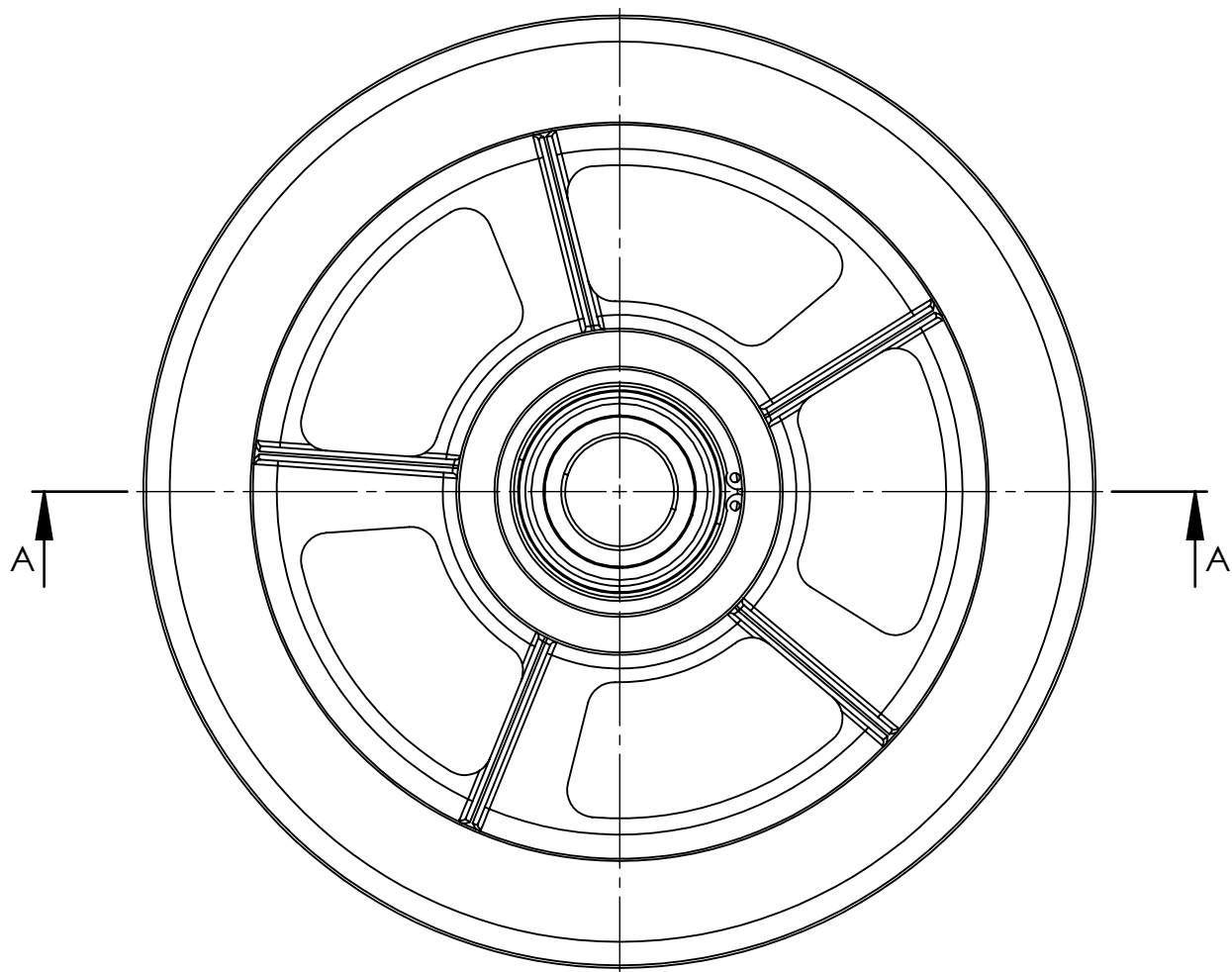
SEZIONE A-A
