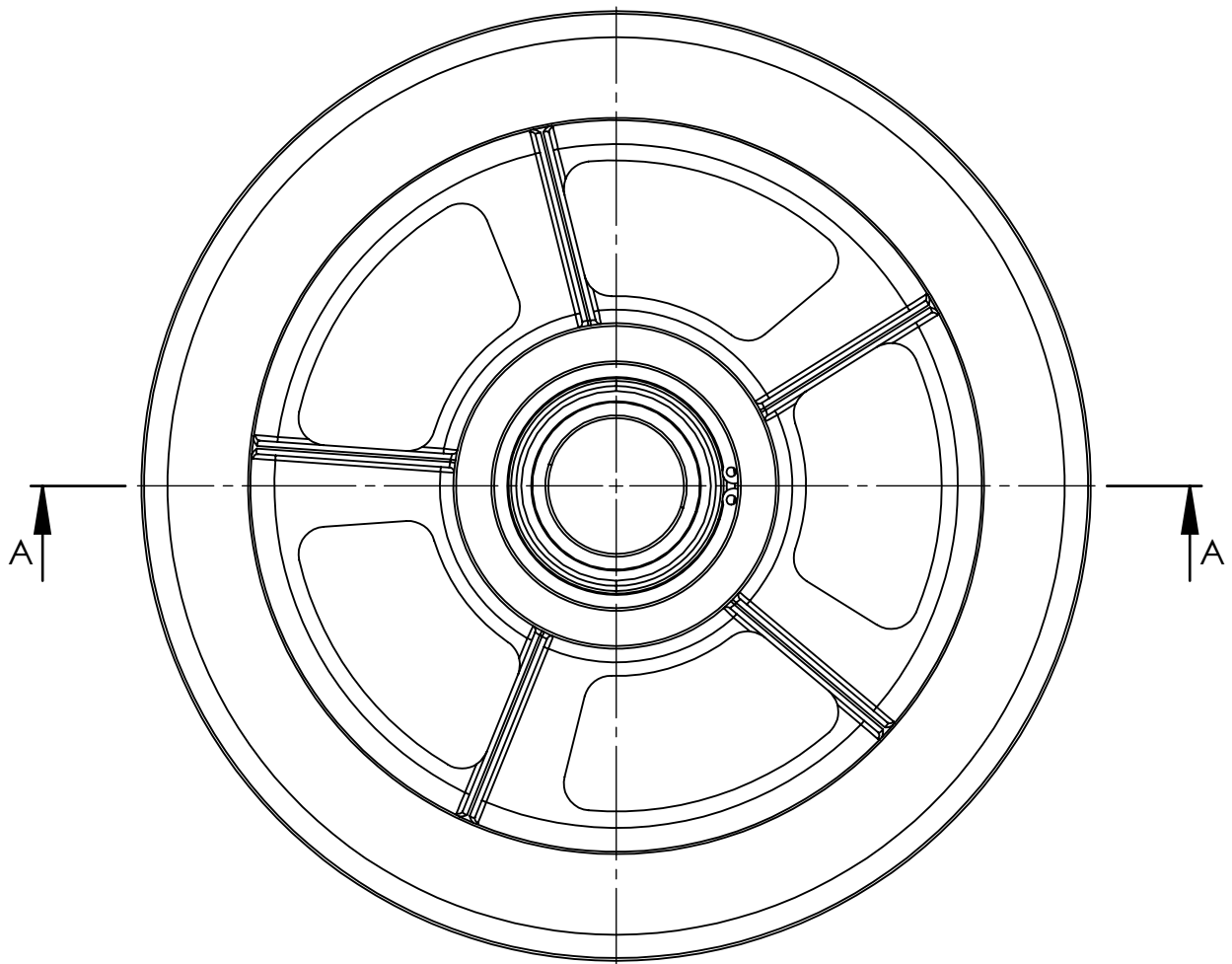
SEZIONE A-A
