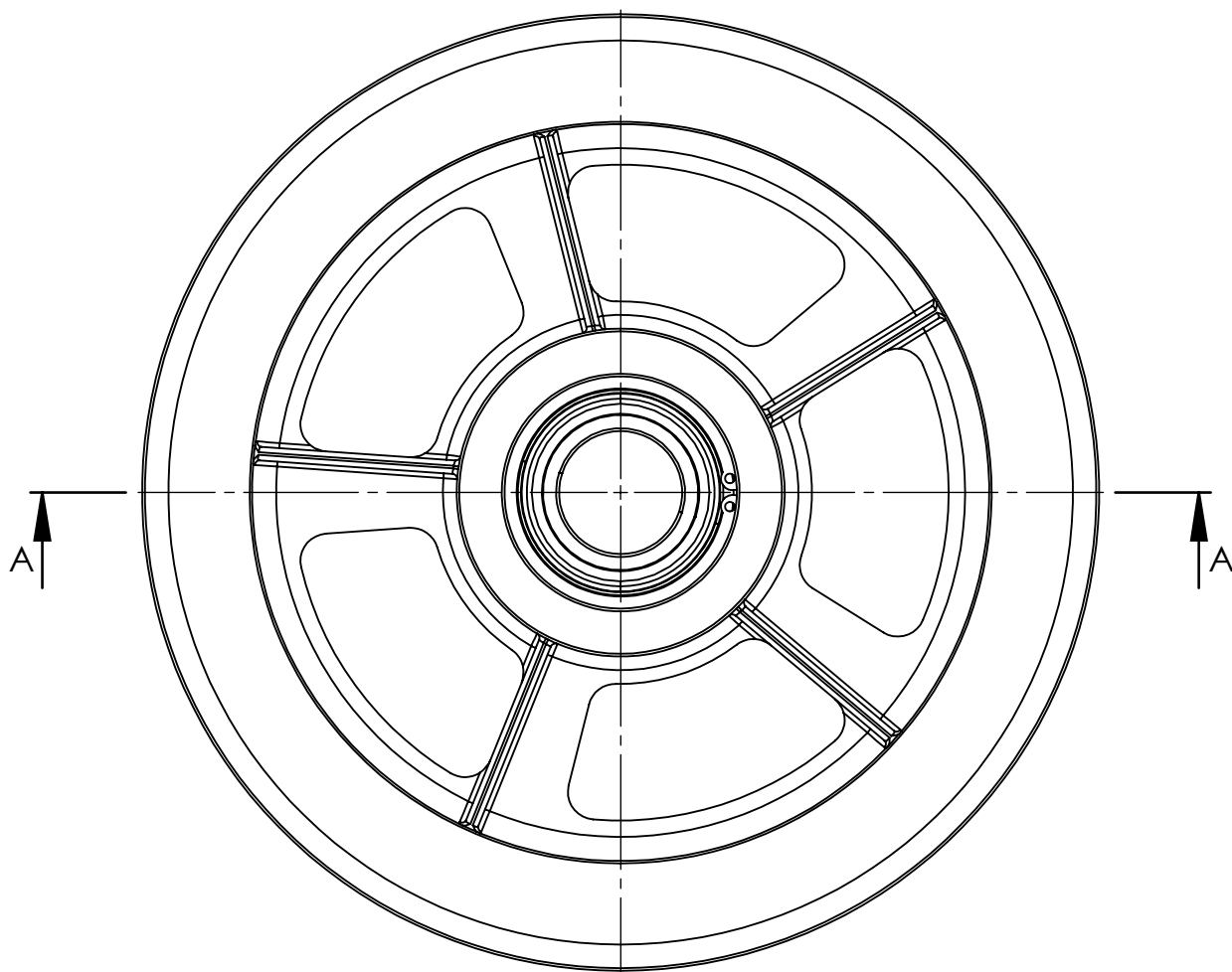
SEZIONE A-A
