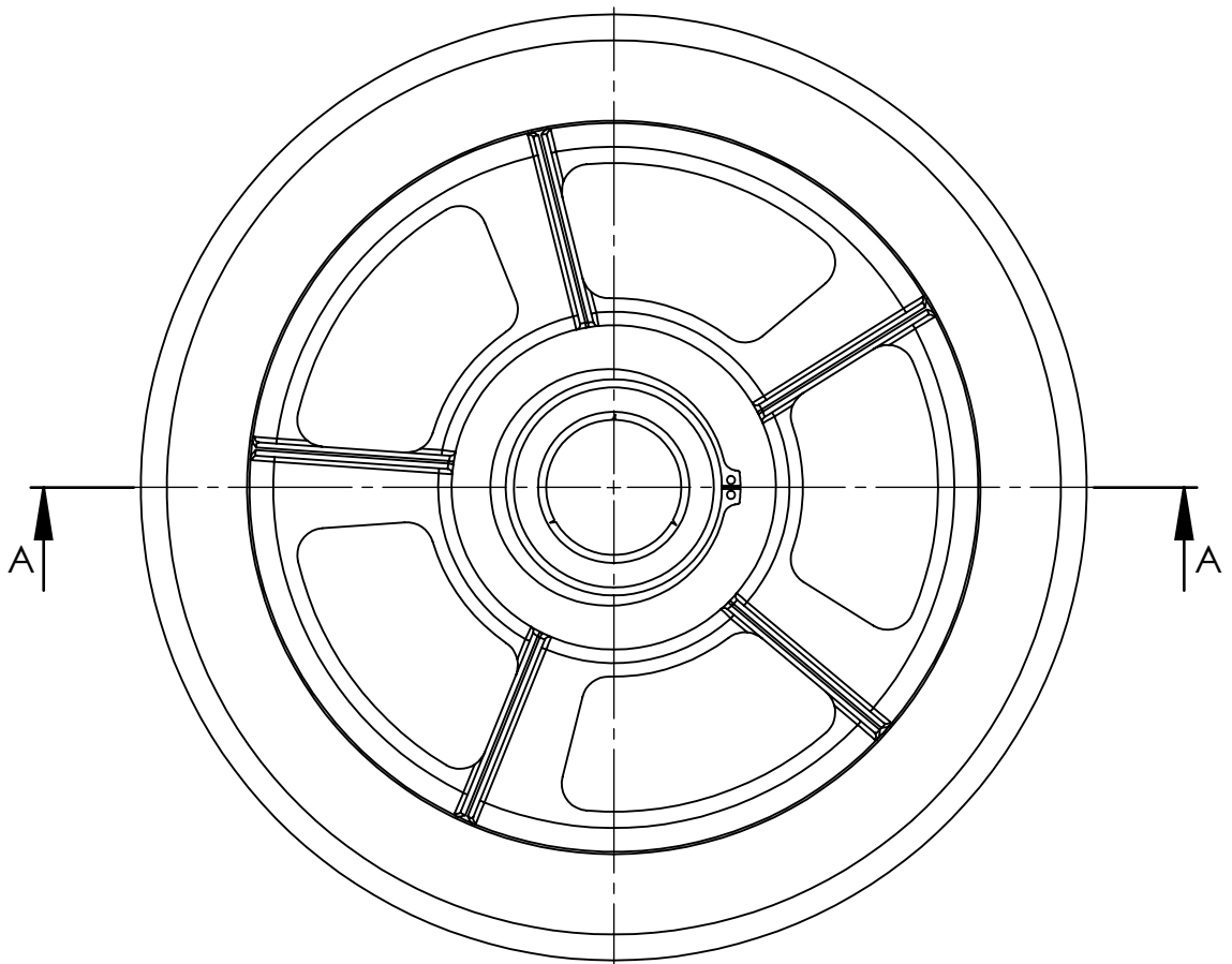
SEZIONE A-A
