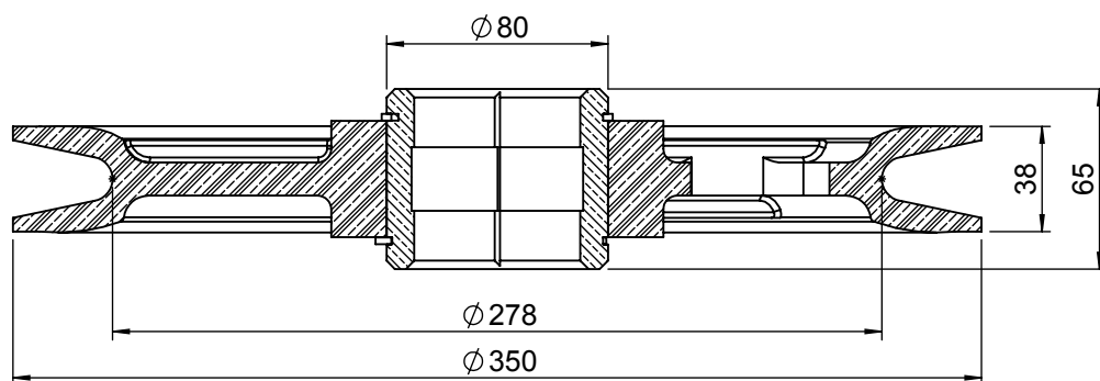
SEZIONE A-A
