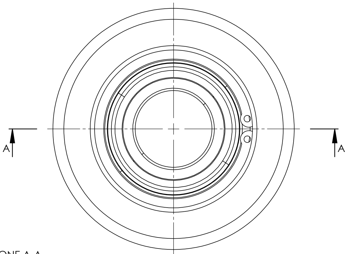
SEZIONE A-A
