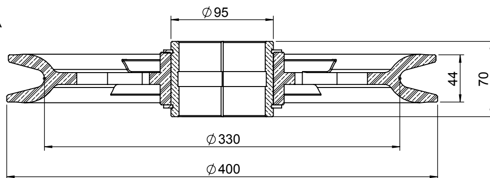
SEZIONE A-A
