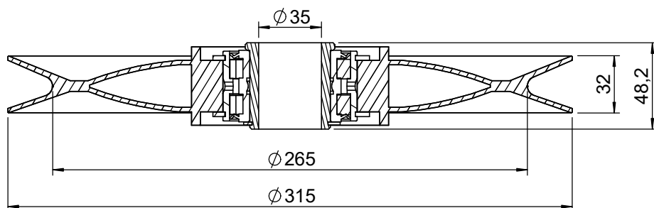
SEZIONE A-A
