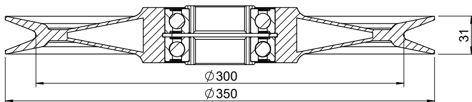
SEZIONE A-A SCALA 1 : 3
