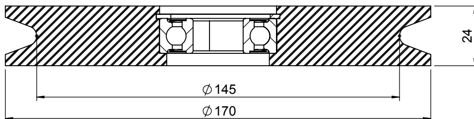
SEZIONE A-A
