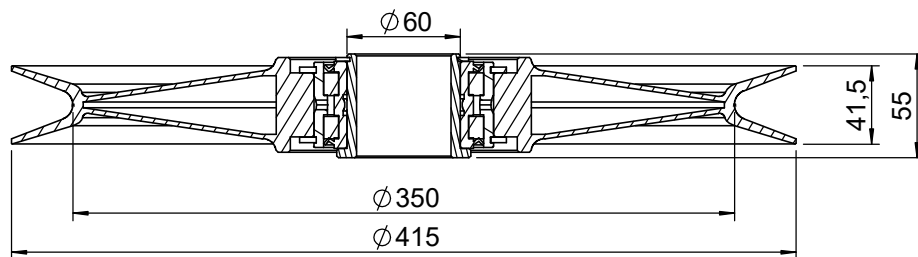
SEZIONE A-A
