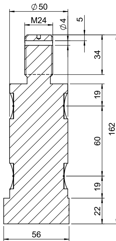
SEZIONE A-A
