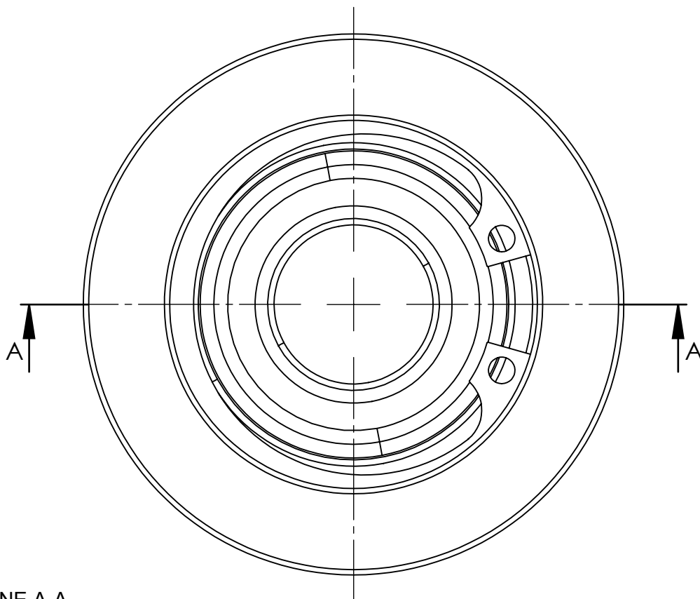
SEZIONE A-A
