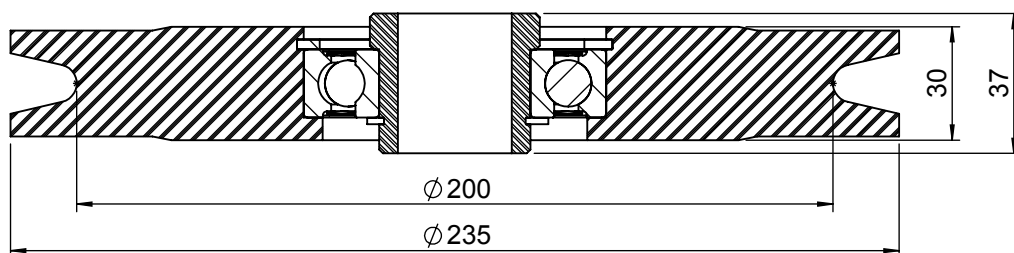
SEZIONE A-A
