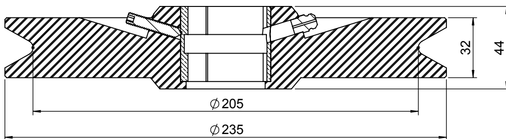
SEZIONE A-A
