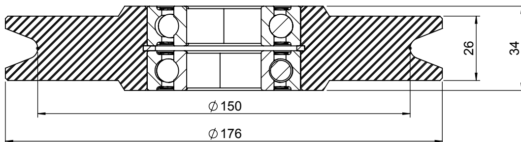
SEZIONE A-A
