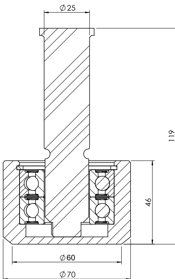
SEZIONE A-A
