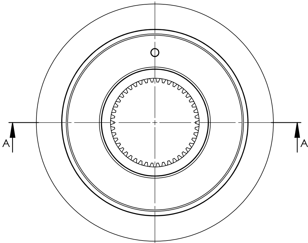
SEZIONE A-A
