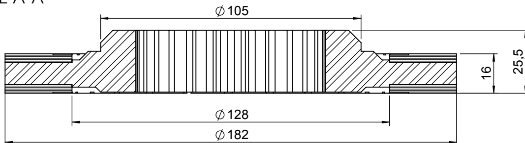
SEZIONE A-A
