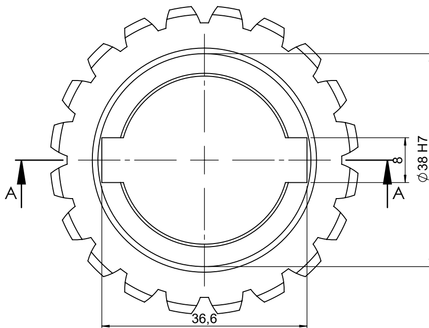
SEZIONE A-A
