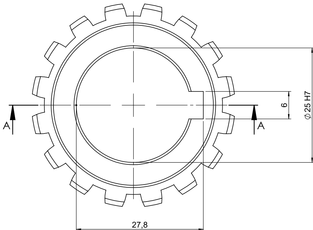
SEZIONE A-A
