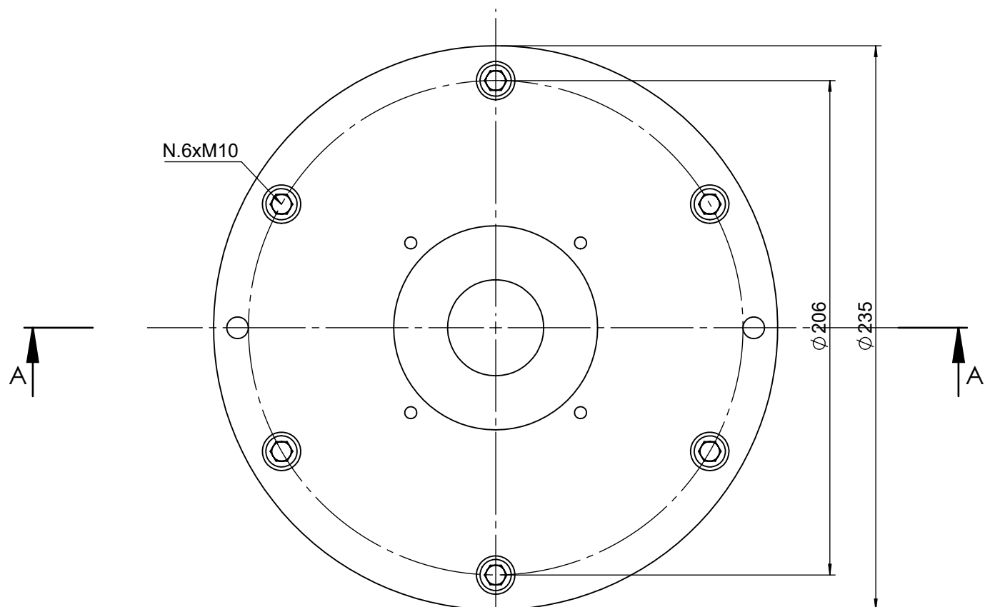
SEZIONE A-A
