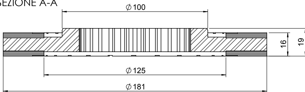
SEZIONE A-A
