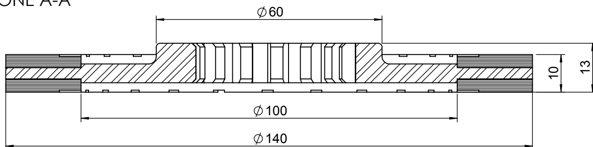
SEZIONE A-A
