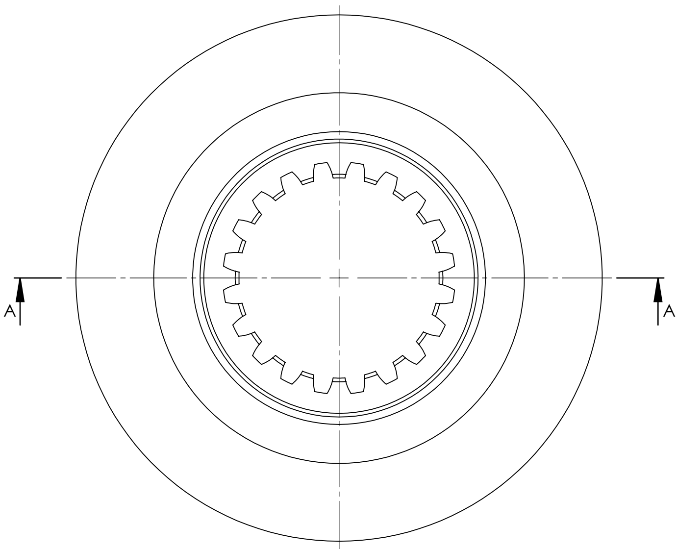
SEZIONE A-A
