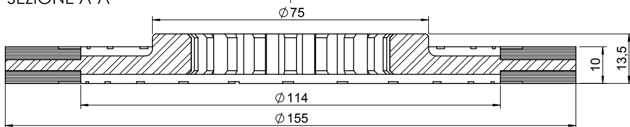
SEZIONE A-A
