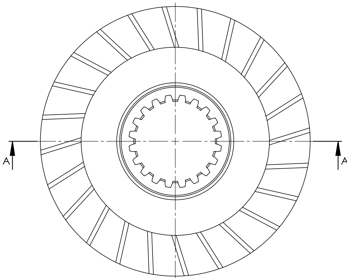
SEZIONE A-A
