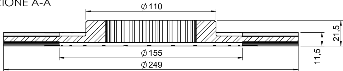
SEZIONE A-A
