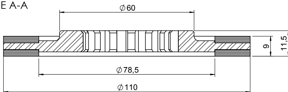
SEZIONE A-A
