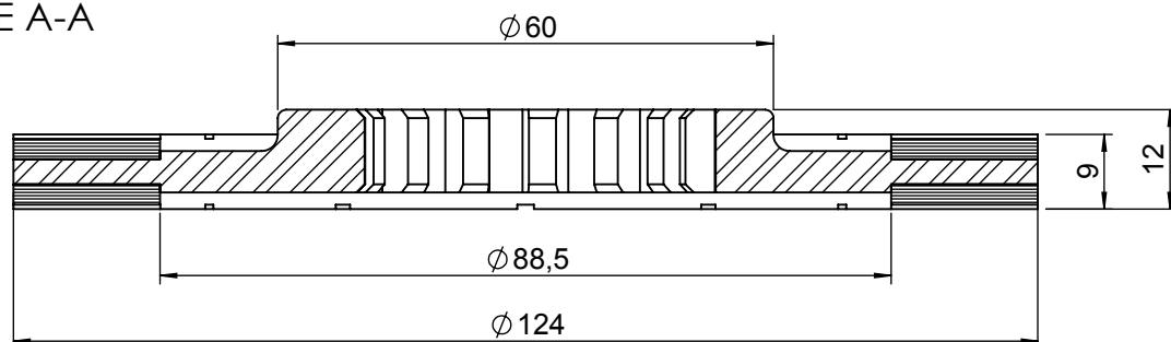
SEZIONE A-A
