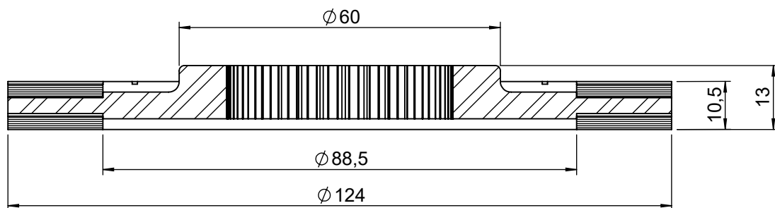
SEZIONE A-A
