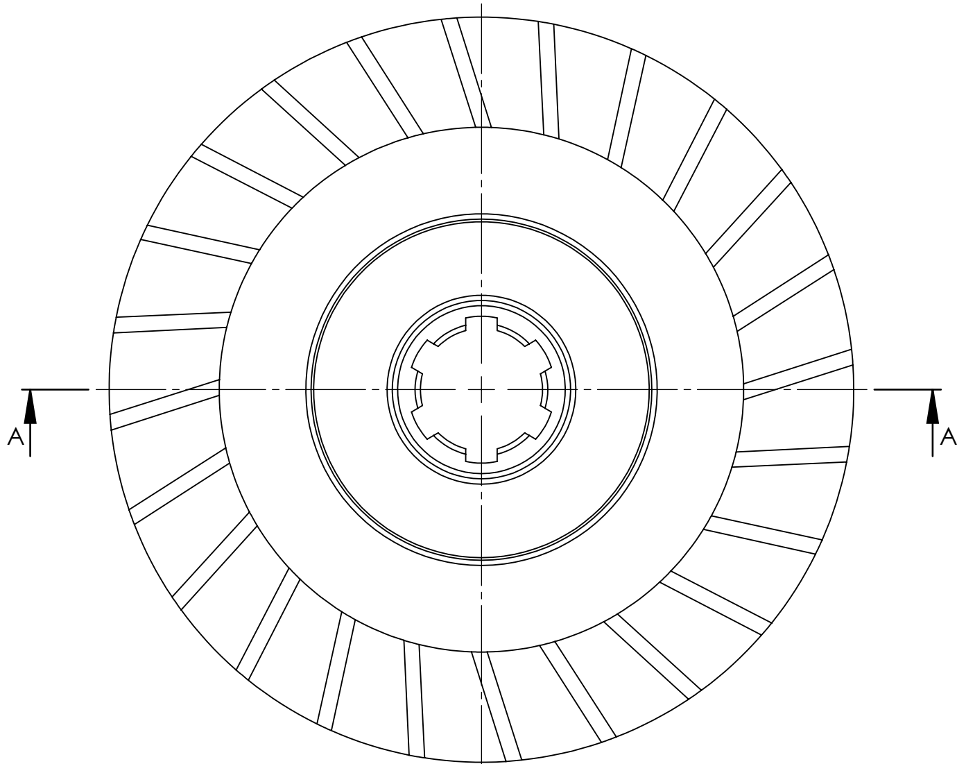
SEZIONE A-A
